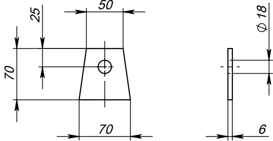
Поз.7 (Проушина)
