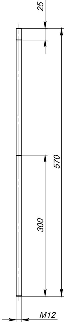
Поз.5 (Шпилька)
